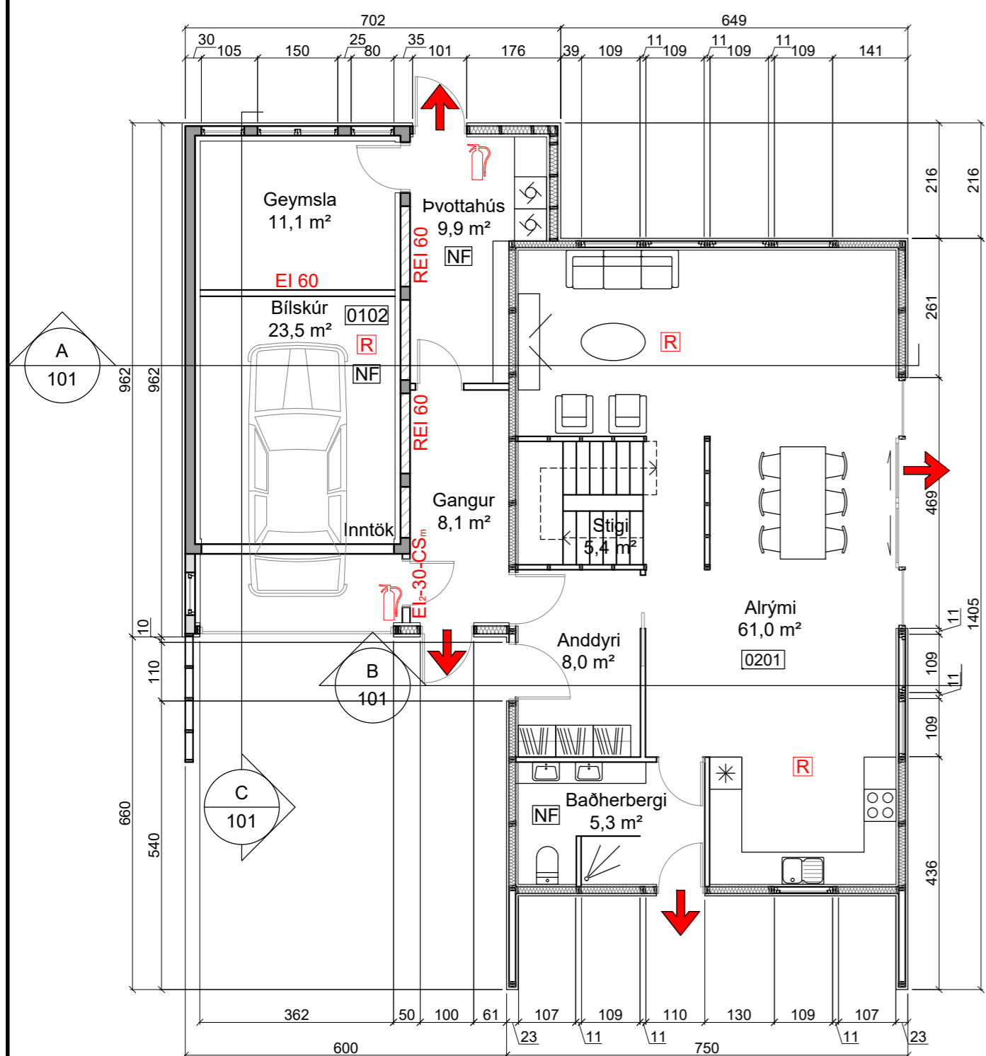
Grunnmynd 1. hæðar, 1:100
