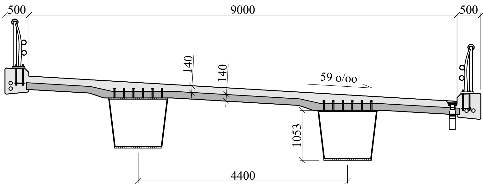
SNIÐ Í HAFI (horft í hækkandi stöð) 1:50
