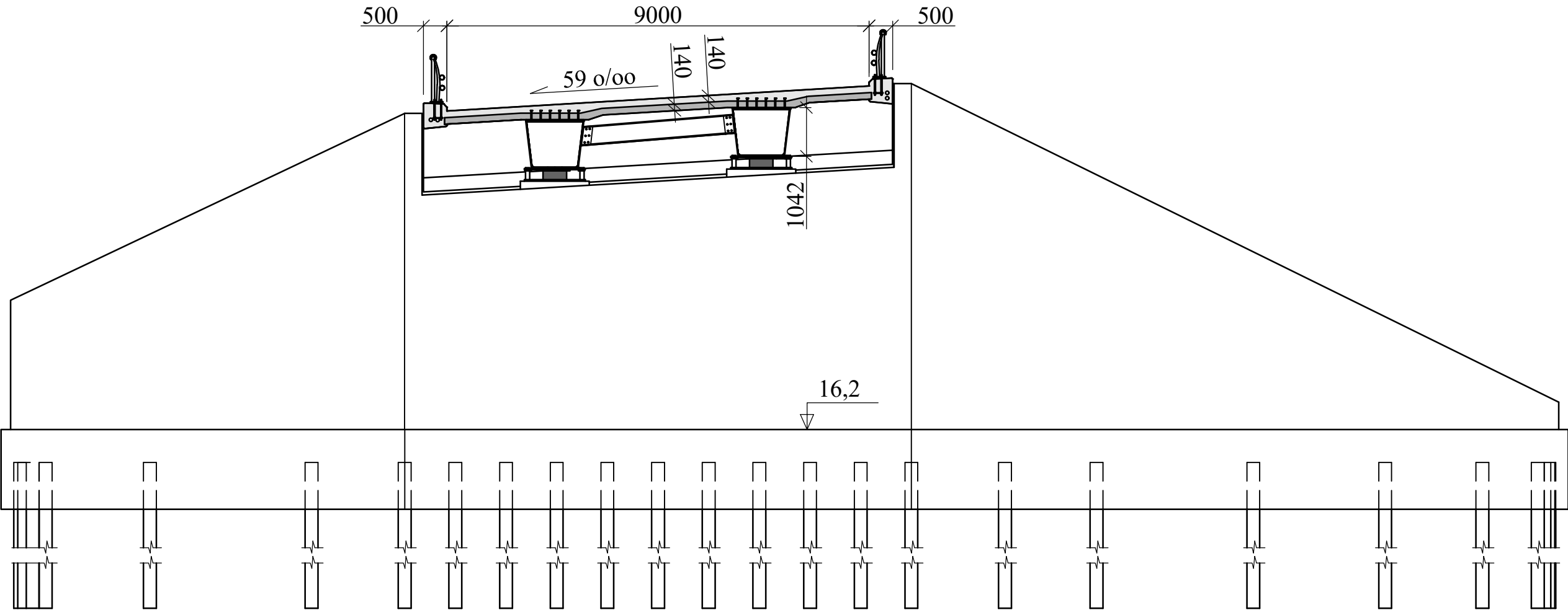
SNIÐ FYRIR FRAMAN EYSTRÍ LANDSTÖPUL 1:100
